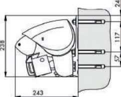
Face-fix
